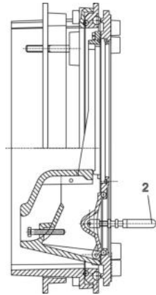
Abb. 7: Stellung 3
