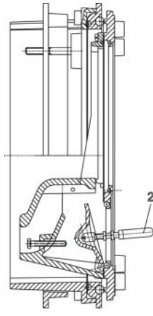
Abb. 6: Stellung 2
