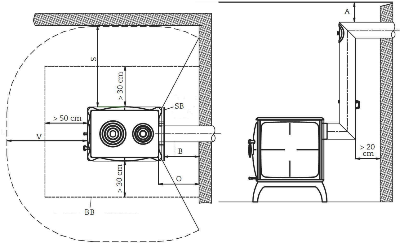
Abb. 6: Erforderliche Abstände der Iron Dog 01 - Iron Dog 05
