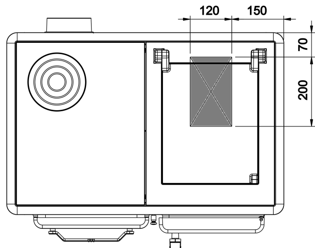
Abb. 5: Verbrennungsluftzuführung
