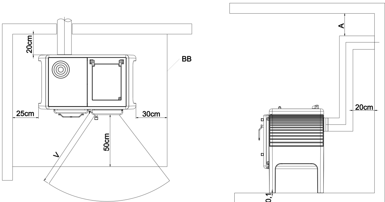
Abb. 7: Erforderliche Abstände für den Iron Dog 06
