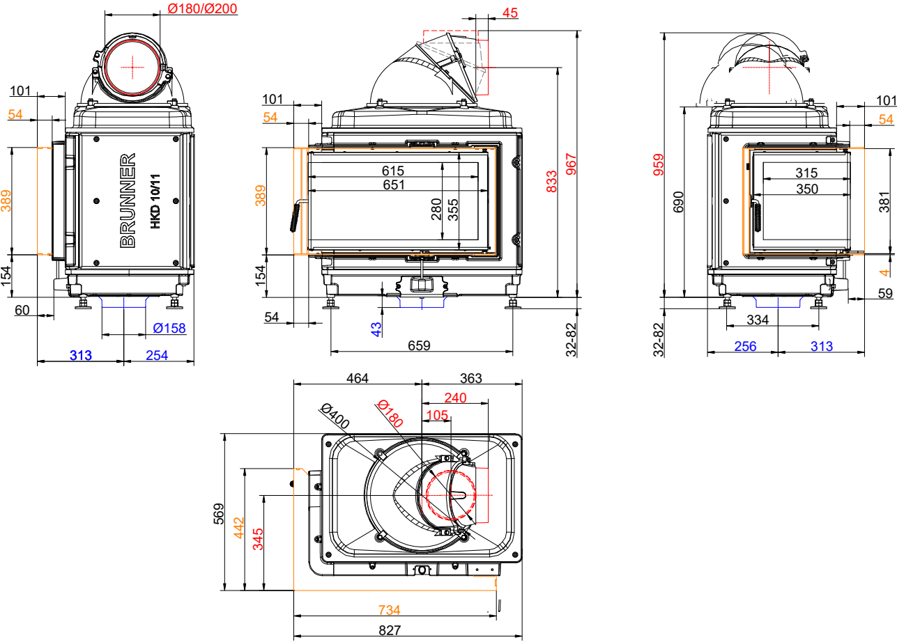
... links mit Gusskuppel, Anbaurahmen
