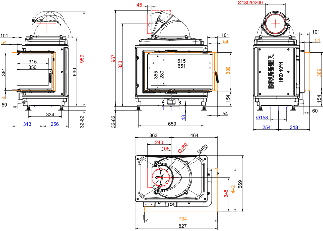
... rechts mit Gusskuppel, Anbaurahmen
