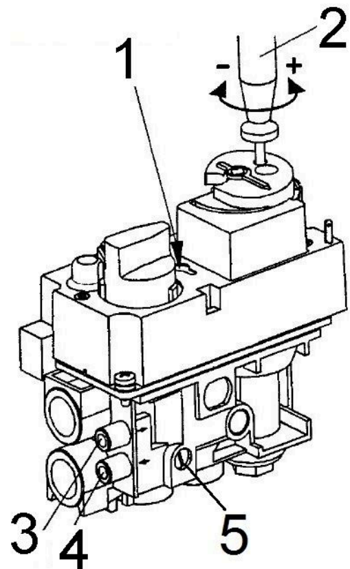
Abb. 8: Gasregelblock
